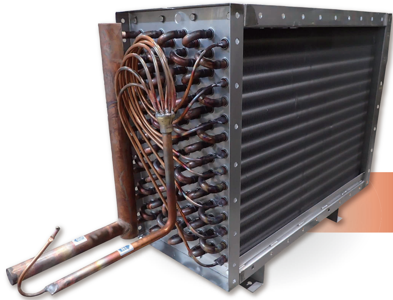
【直膨用コイルプレートフィンチューブ型】
