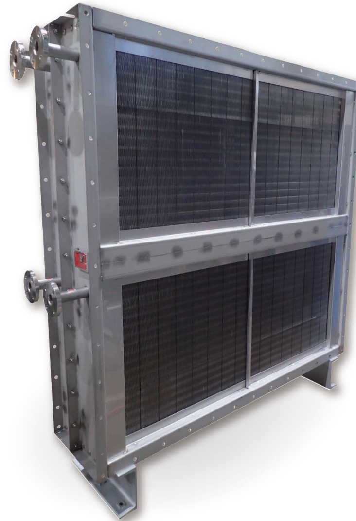
【乾燥炉用蒸気ヒーター上下分割型】
