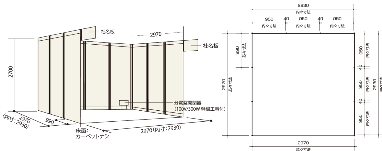
システムパネル壁面形状
