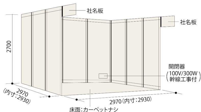
システムパネル壁面形状
